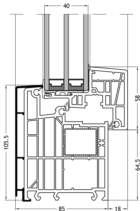
Aro em forma de Z 964N com folha Nova-line 953
