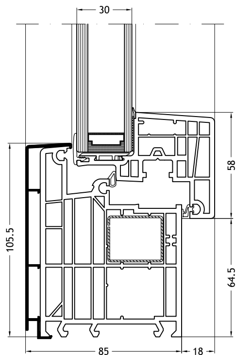
Aro em forma de Z 964N com folha Nova-line 971
