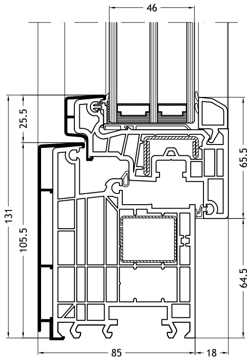
Blendrahmen L-Form 963N mit Flügel Slim-line
