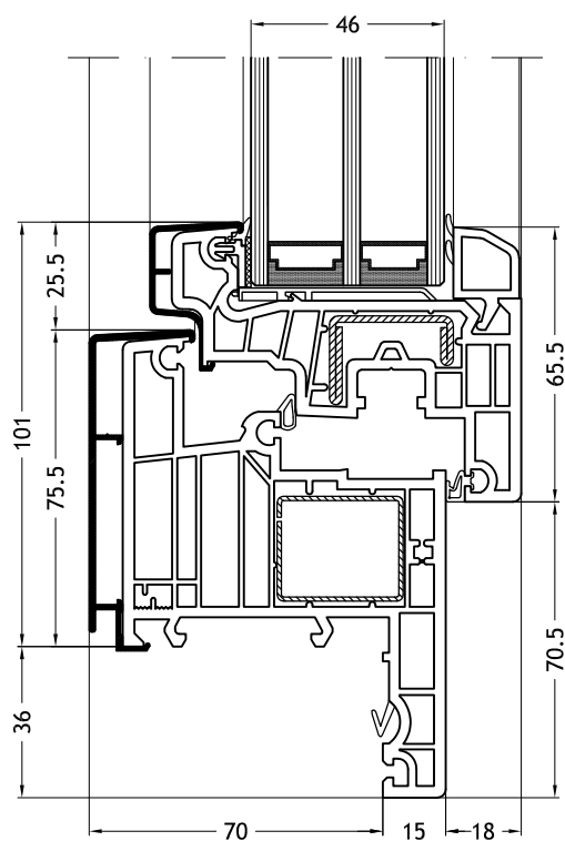
Telaio a Z 967N con anta Slim-line
