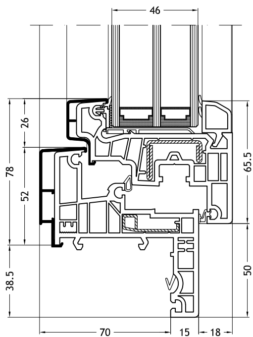
Marco Z - 965N con hoja Slim-line
