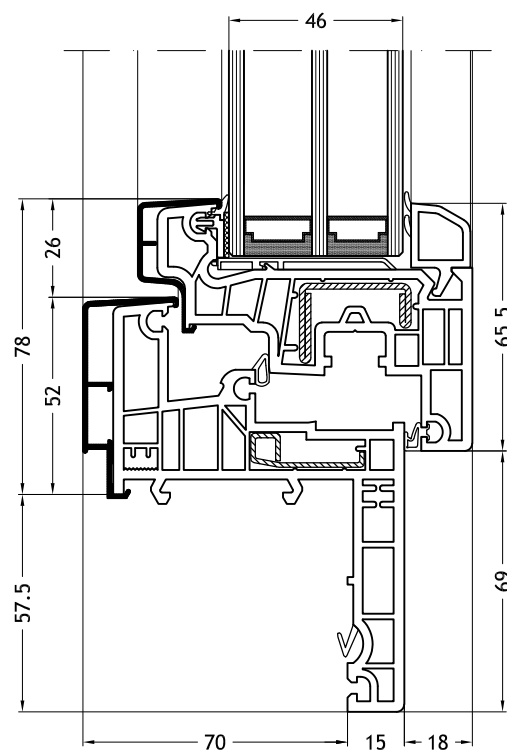
Marco Z - 966N con hoja Slim-line
