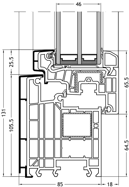
Marco L - 963N con hoja Slim-line
