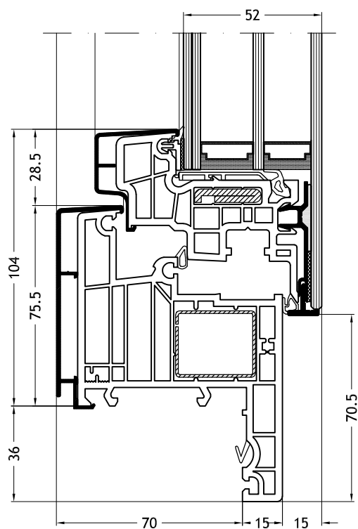
Telaio a Z 967N con anta Slim-line Cristal
