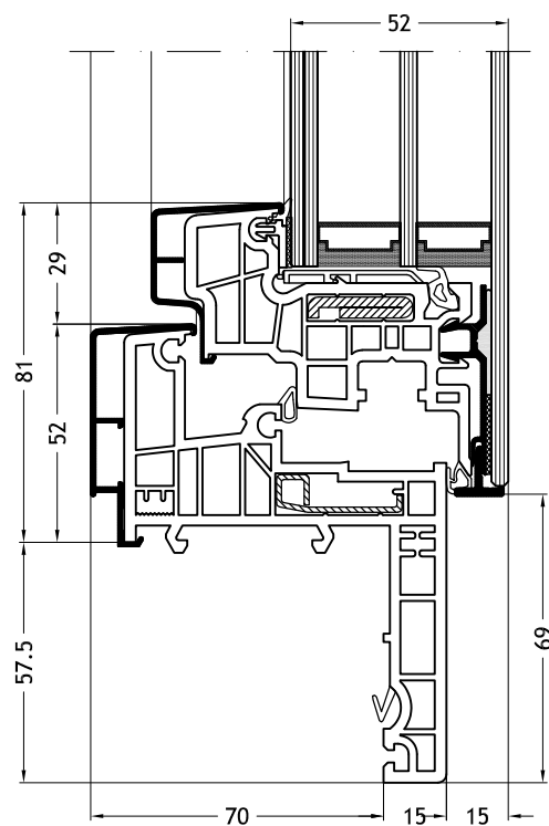
Dormant en Z, 966N avec ouvrant Slim-line Cristal
