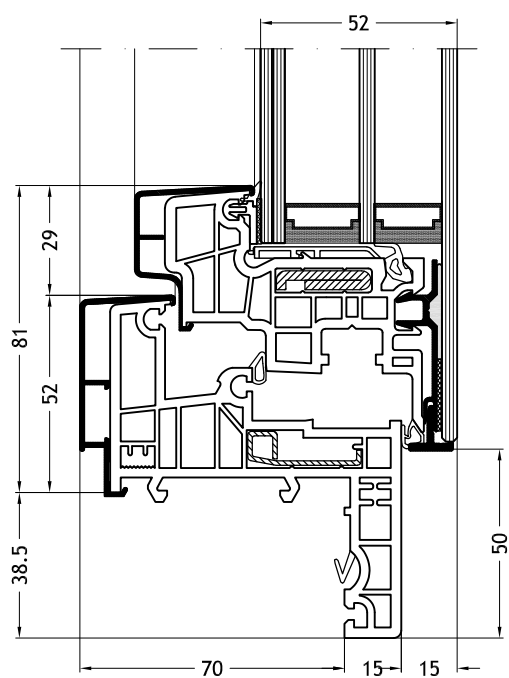
Dormant en Z, 965N avec ouvrant Slim-line Cristal
