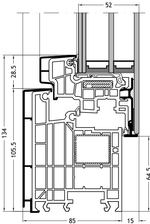
Marco L - 963N con hoja Slim-line Cristal
