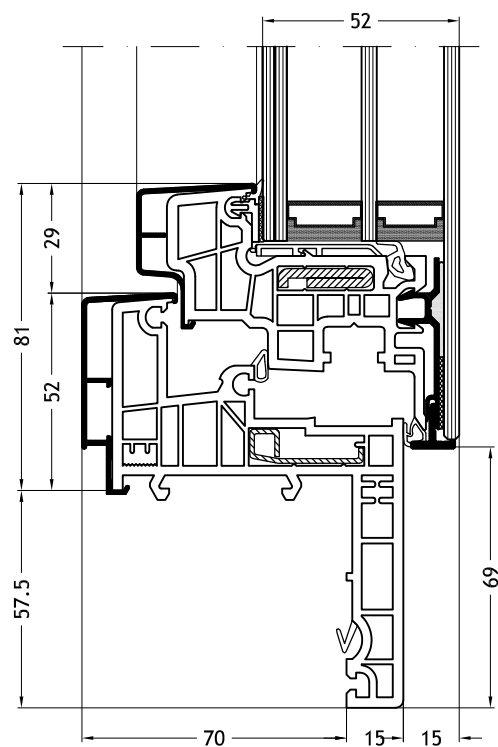
Kozijn Z-vorm 966N met vleugel Slim-line Cristal
