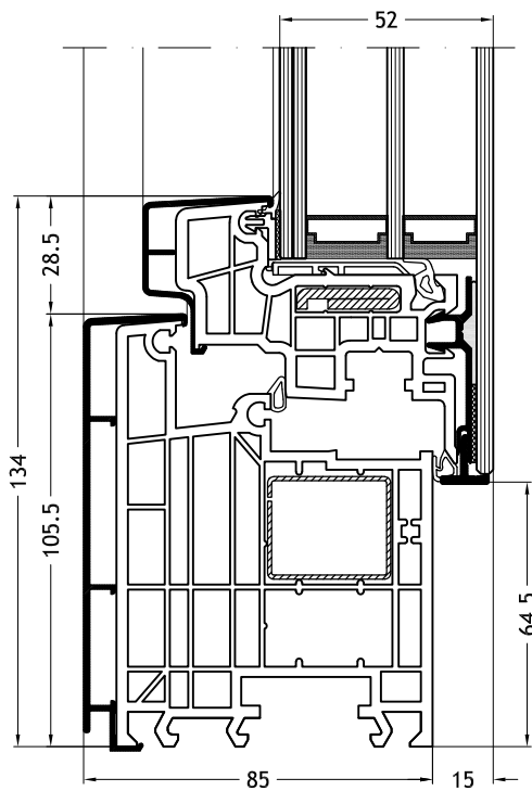
Kozijn L-vorm 963N met vleugel Slim-line Cristal
