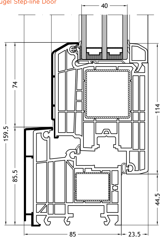
Blendrahmen L-Form 962N mit Flügel Step-line Door
