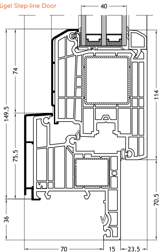
Blendrahmen Z-Form 967N mit Flügel Step-line Door
