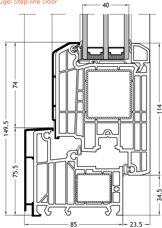
Blendrahmen L-Form 961N mit Flügel Step-line Door
