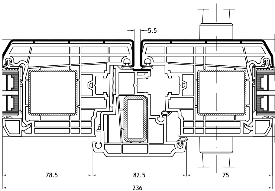
Klassische Stulp-Mittelpartie A28K mit Flügel Step-line Door out
