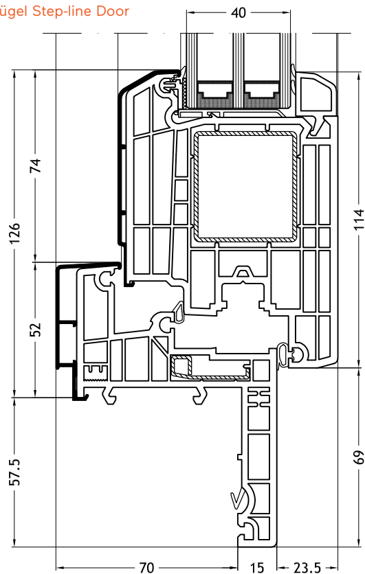
Blendrahmen Z-Form 966N mit Flügel Step-line Door
