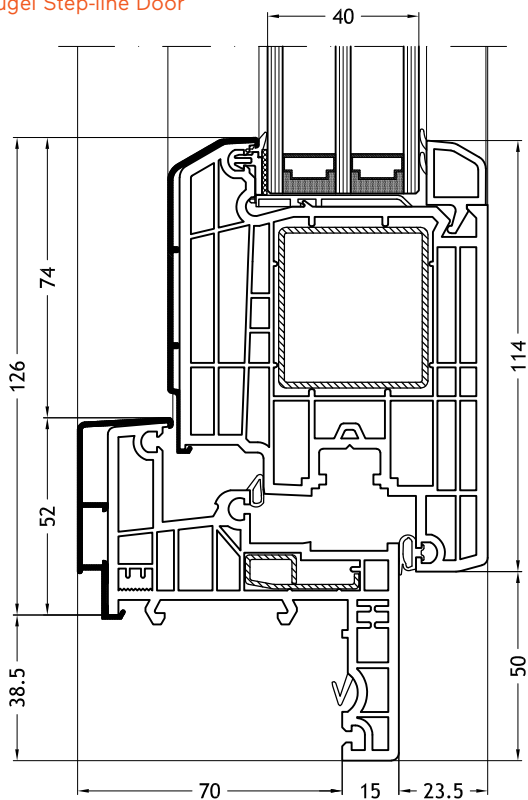
Blendrahmen Z-Form 965N mit Flügel Step-line Door
