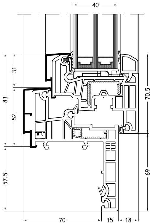
Blendrahmen Z-Form 966N mit Flügel Step-line
