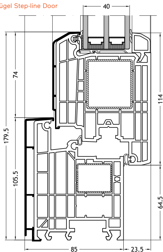
Blendrahmen L-Form 963N mit Flügel Step-line Door
