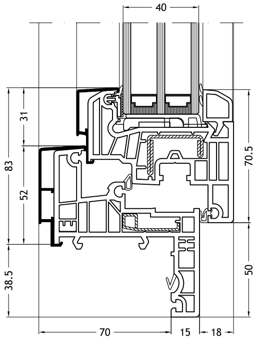
Blendrahmen Z-Form 965N mit Flügel Step-line
