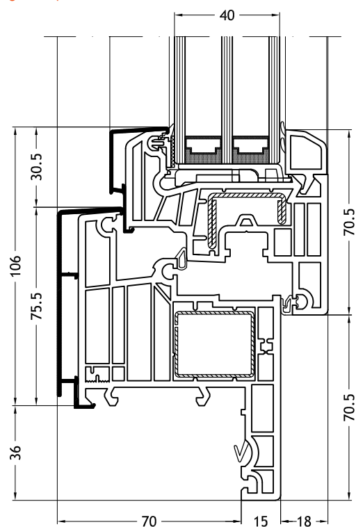
Blendrahmen Z-Form 967N mit Flügel Step-line
