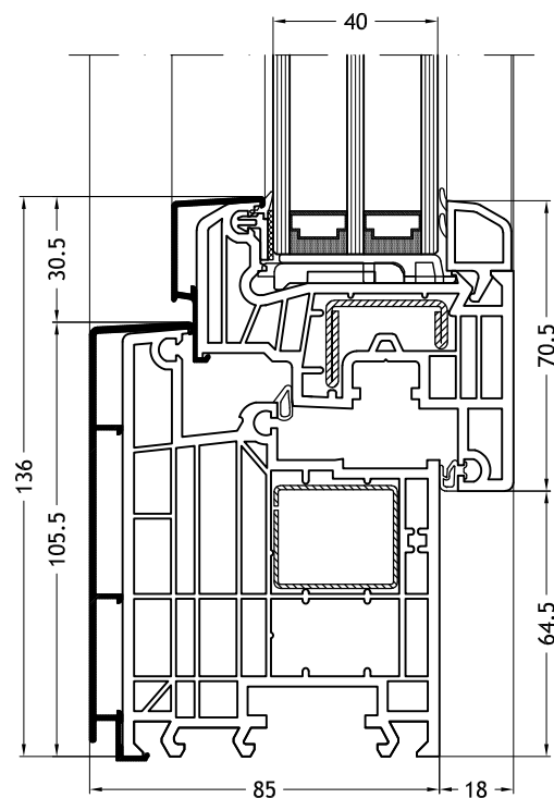
Blendrahmen L-Form 963N mit Flügel Step-line
