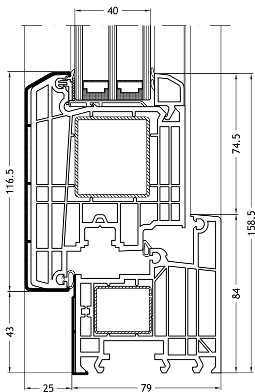
Blendrahmen L-Form A9620K mit Flügel Step-line Door out
