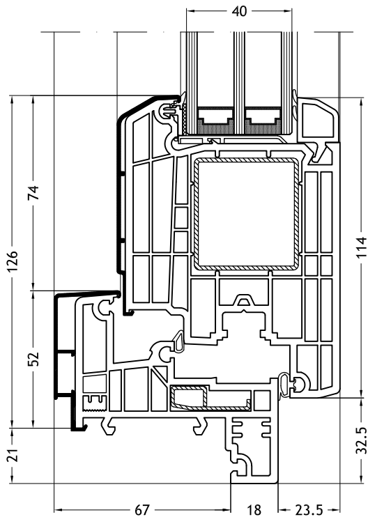
Blendrahmen Z-Form 964N mit Flügel Step-line Door
