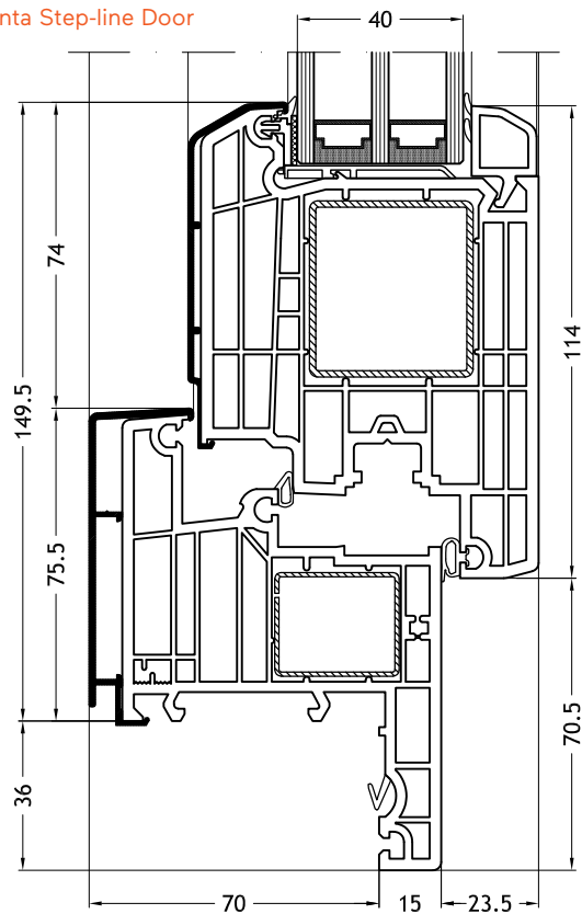
Telaio a Z 967N con anta Step-line Door
