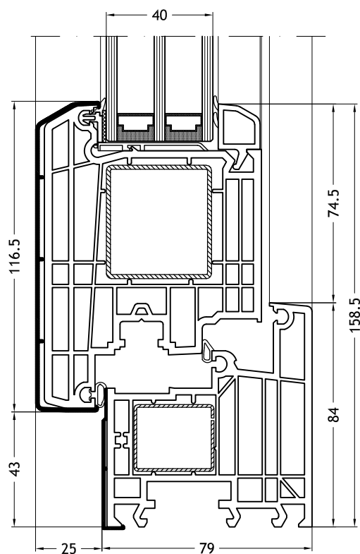
Telaio a L A9620K con anta Step-line Door out
