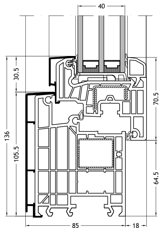
Telaio a L 963N con anta Step-line
