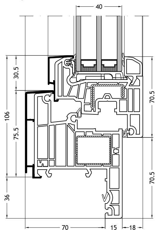
Telaio a Z 967N con anta Step-line
