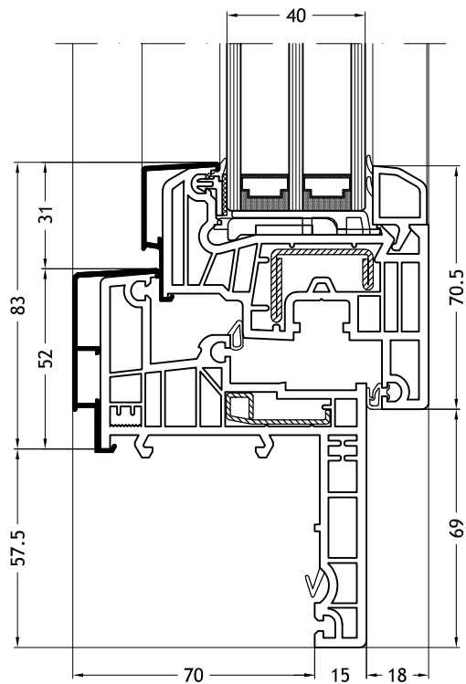
Telaio a Z 966N con anta Step-line
