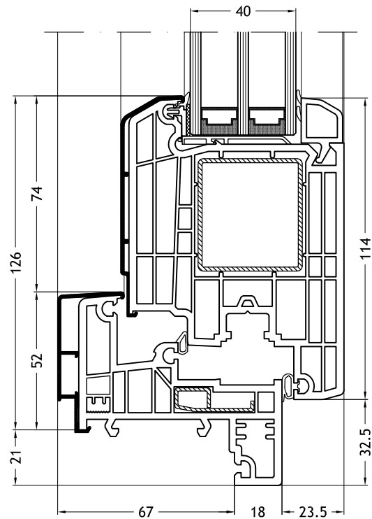
Telaio a Z 964N con anta Step-line Door
