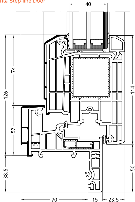
Telaio a Z 965N con anta Step-line Door
