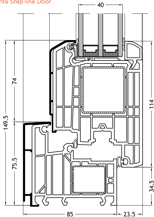
Telaio a L 961N con anta Step-line Door
