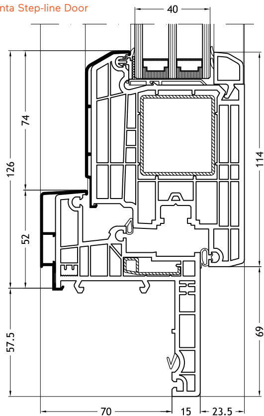
Telaio a Z 966N con anta Step-line Door
