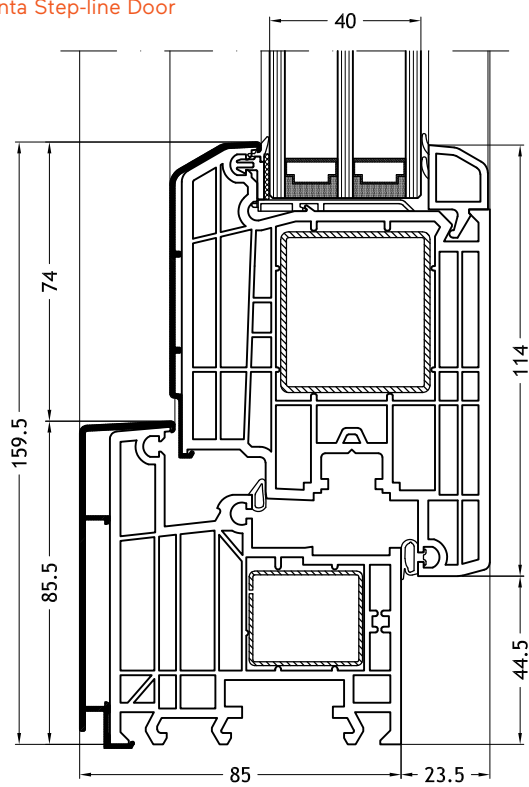
Telaio a L 962N con anta Step-line Door
