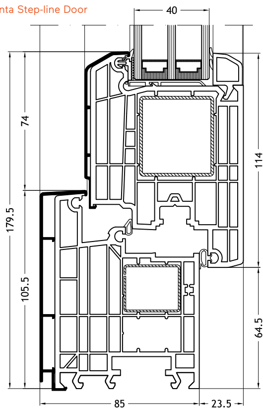
Telaio a L 963N con anta Step-line Door
