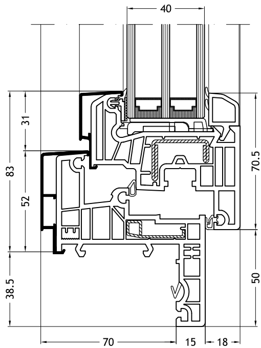
Telaio a Z 965N con anta Step-line
