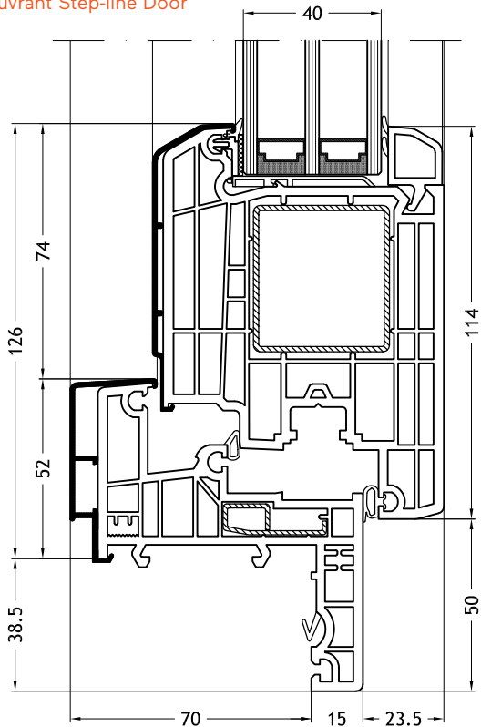
Dormant en Z, 965N avec ouvrant Step-line Door
