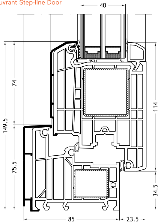
Dormant en L, 961N avec ouvrant Step-line Door
