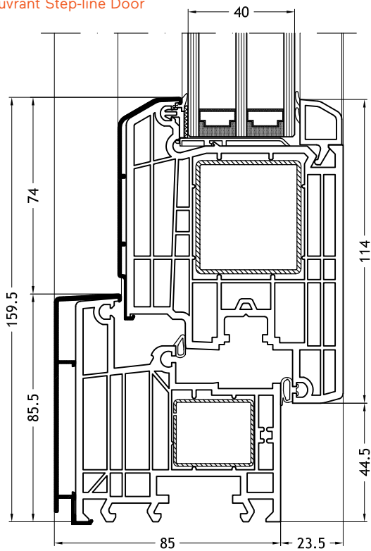
Dormant en L, 962N avec ouvrant Step-line Door
