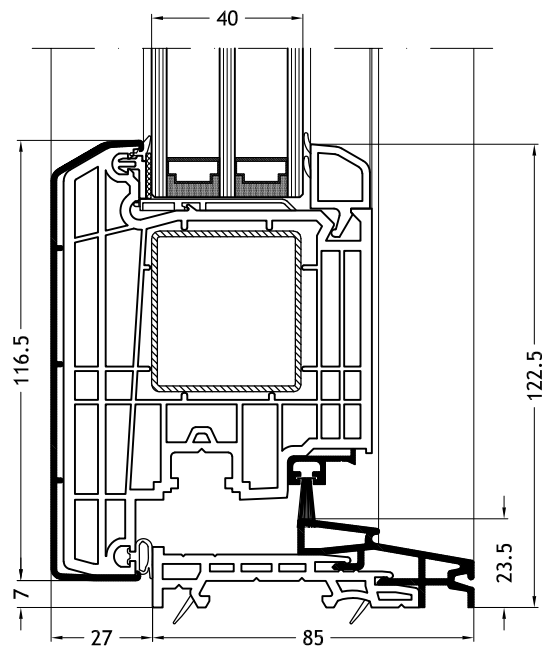
Seuil plat avec ouvrant Step-line Door out
