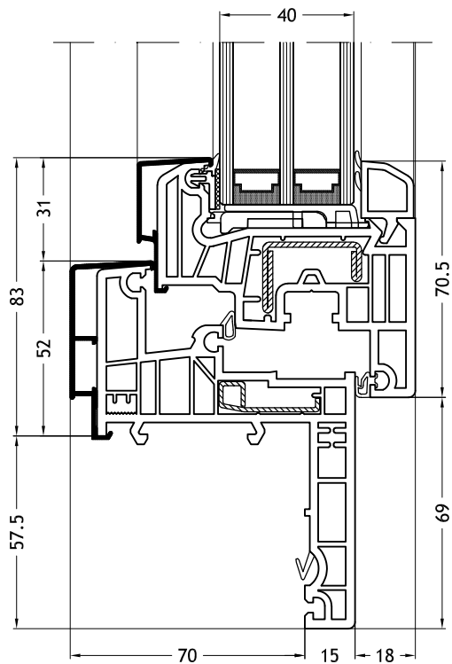
Dormant en Z, 966N avec ouvrant Step-line
