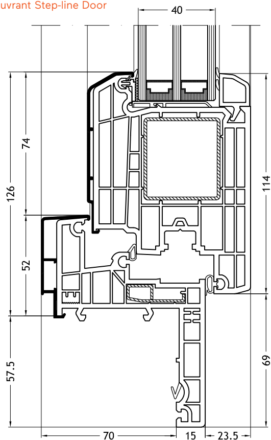
Dormant en Z, 966N avec ouvrant Step-line Door
