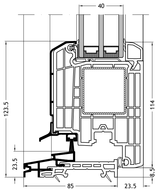
Seuil plat avec ouvrant Step-line Door
