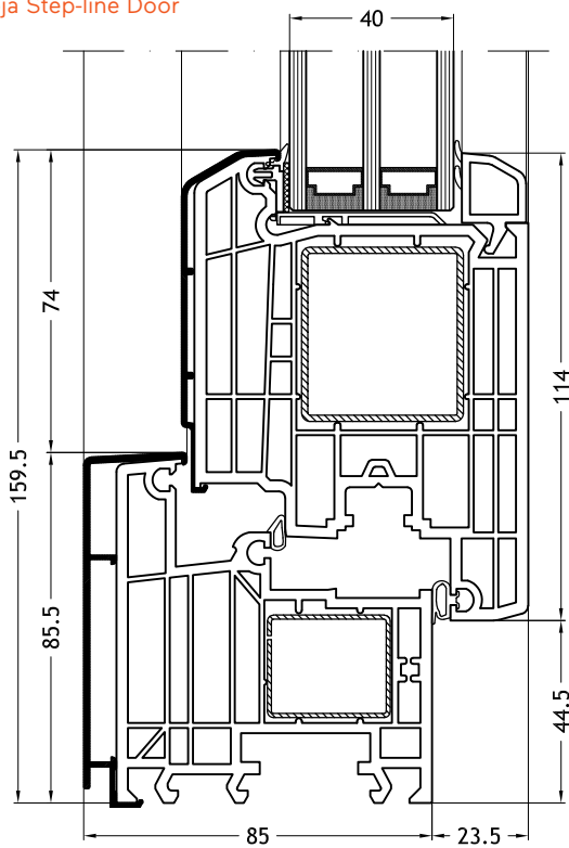
Marco L - 962N con hoja Step-line Door
