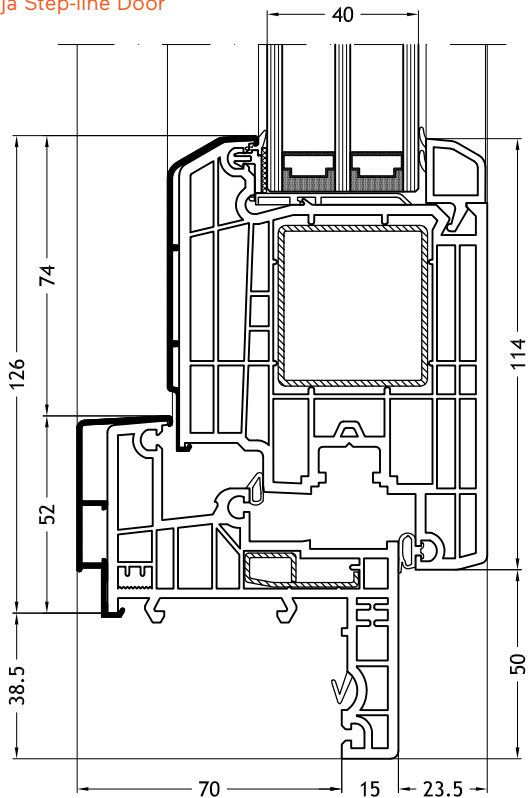
Marco Z - 965N con hoja Step-line Door
