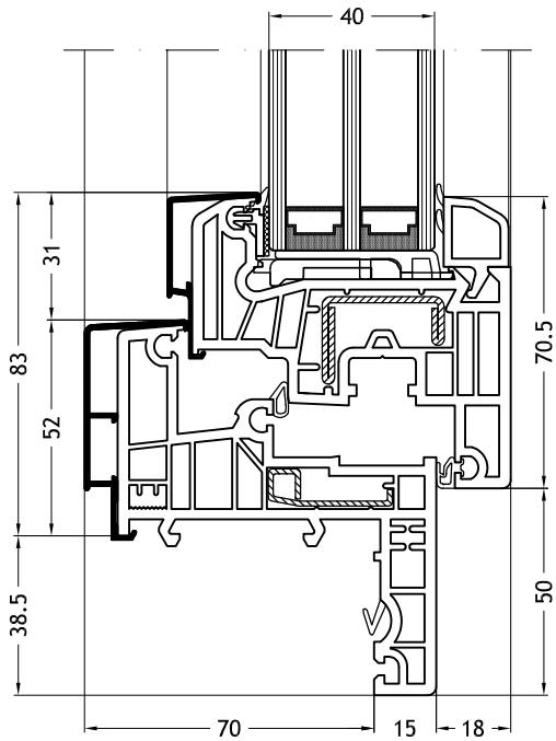
Marco Z - 965N con hoja Step-line
