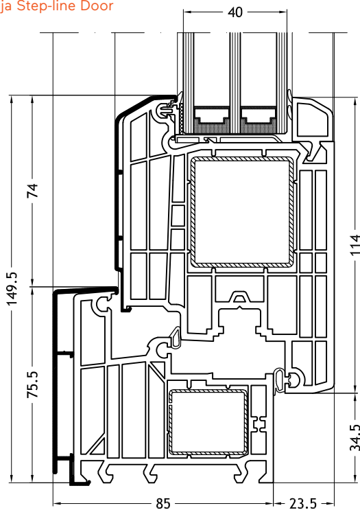
Marco L - 961N con hoja Step-line Door
