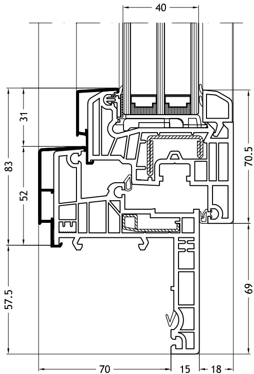
Marco Z - 966N con hoja Step-line
