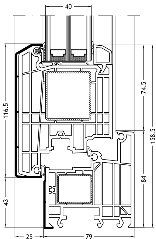
Kozijn L-vorm A9620K met vleugel Step-line Door out
