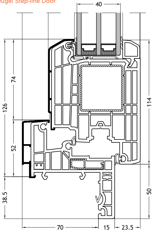
Kozijn Z-vorm 965N met vleugel Step-line Door
