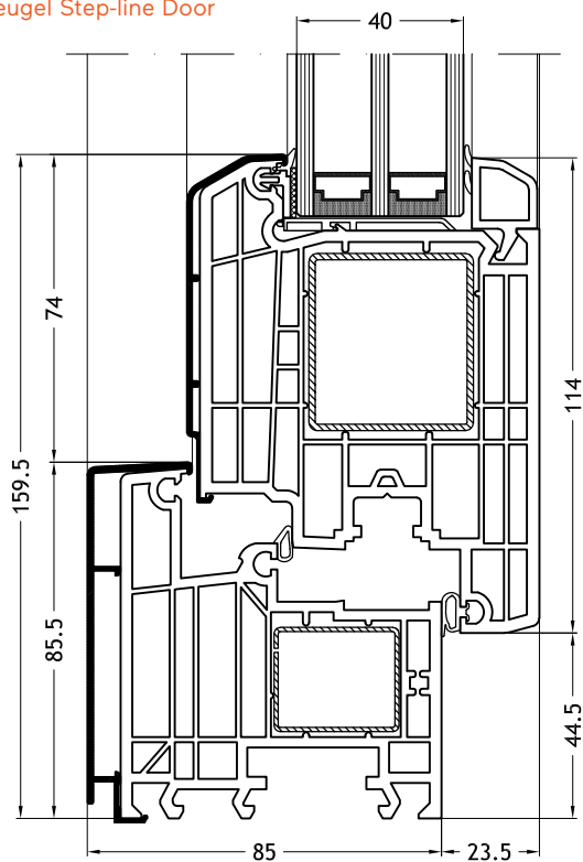
Kozijn L-vorm 962N met vleugel Step-line Door
