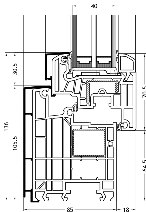
Kozijn L-vorm 963N met vleugel Step-line
