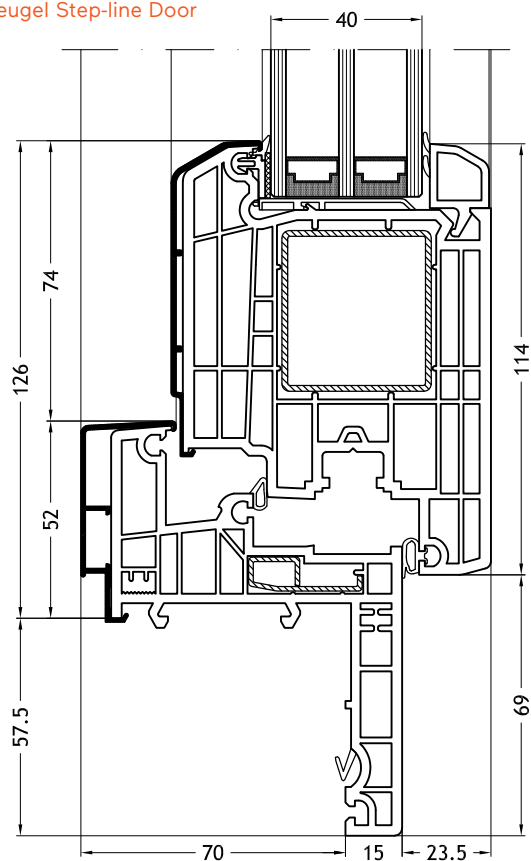
Kozijn Z-vorm 966N met vleugel Step-line Door
