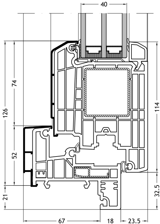
Kozijn Z-vorm 964N met vleugel Step-line Door
