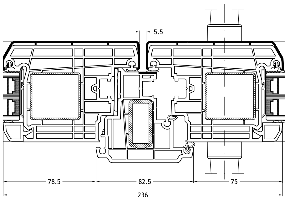
Klassieke stolp-middenpartij A28K met vleugel Step-line Door out
