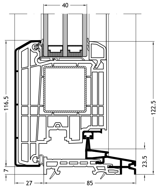
Vlakke onderdorpel met vleugel Step-line Door out
