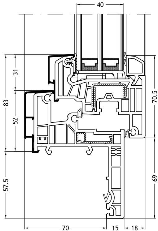
Kozijn Z-vorm 966N met vleugel Step-line
