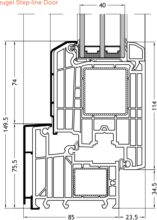
Kozijn L-vorm 961N met vleugel Step-line Door
