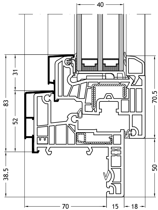
Kozijn Z-vorm 965N met vleugel Step-line
