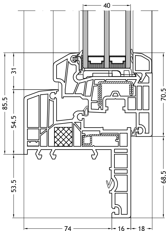
Blendrahmen Z-Form 929 mit Flügel Classic-line
