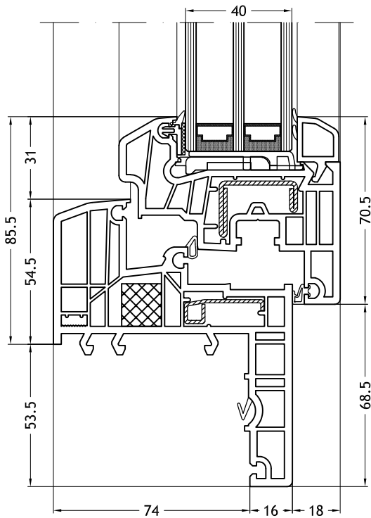
Telaio a Z 929 con anta Classic-line
