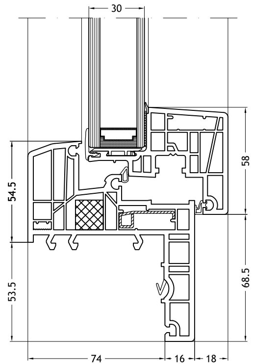
Blendrahmen Z-Form 929 mit Flügel Nova-line 971
