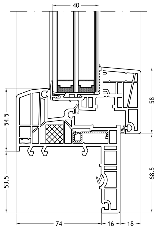
Blendrahmen Z-Form 929 mit Flügel Nova-line 953
