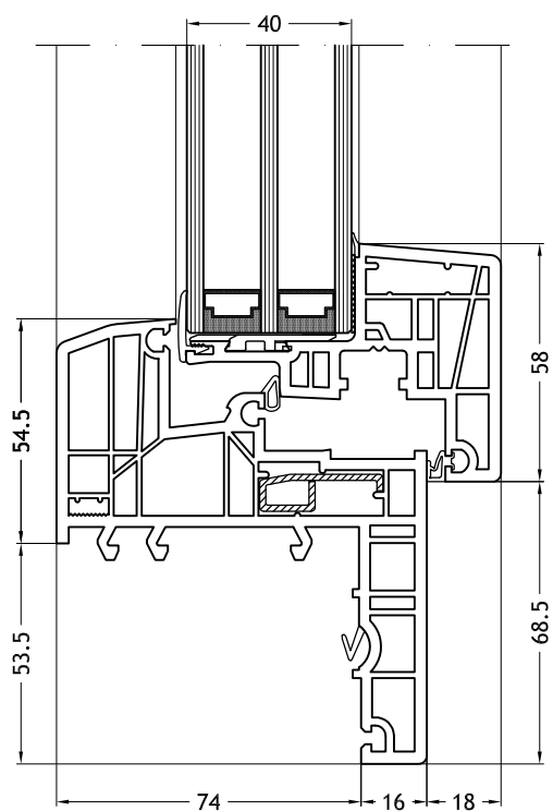
Soleira plana com folha Nova-line 953
