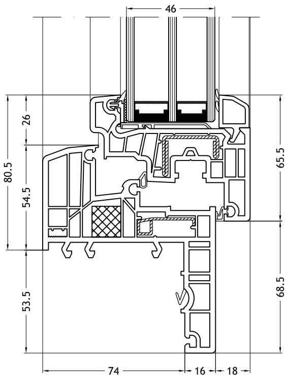
Telaio a Z 929 con anta Slim-line
