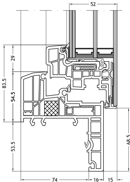
Blendrahmen Z-Form 929 mit Flügel Slim-line Cristal
