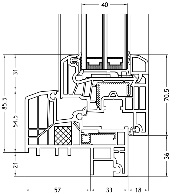
Kozijn Z-vorm 923 met vleugel Step-line
