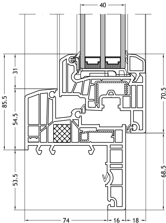
Kozijn Z-vorm 929 met vleugel Step-line
