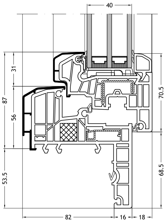
Blendrahmen Z-Form 129K mit Flügel Classic-line C
