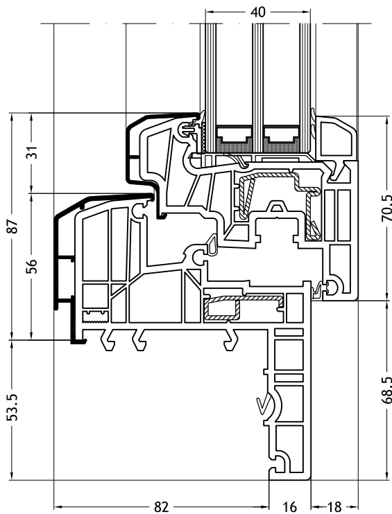
Aro em forma de Z 929K com folha Classic-line C
