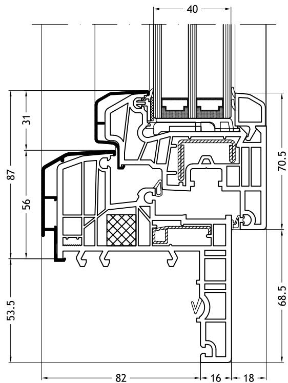
Telaio a Z 129K con anta Classic-line C
