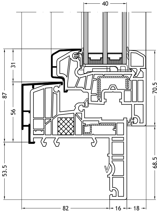
Telaio a Z 129N con anta Classic-line N
