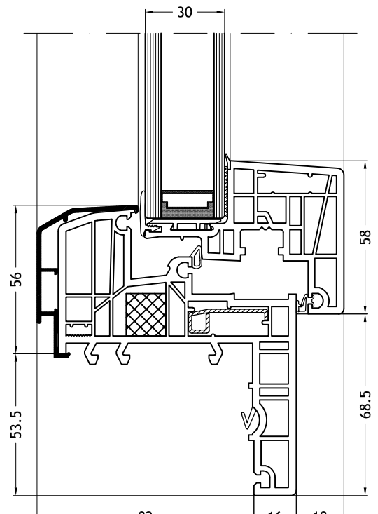
Flache Schwelle mit Flügel Nova-line C 971
