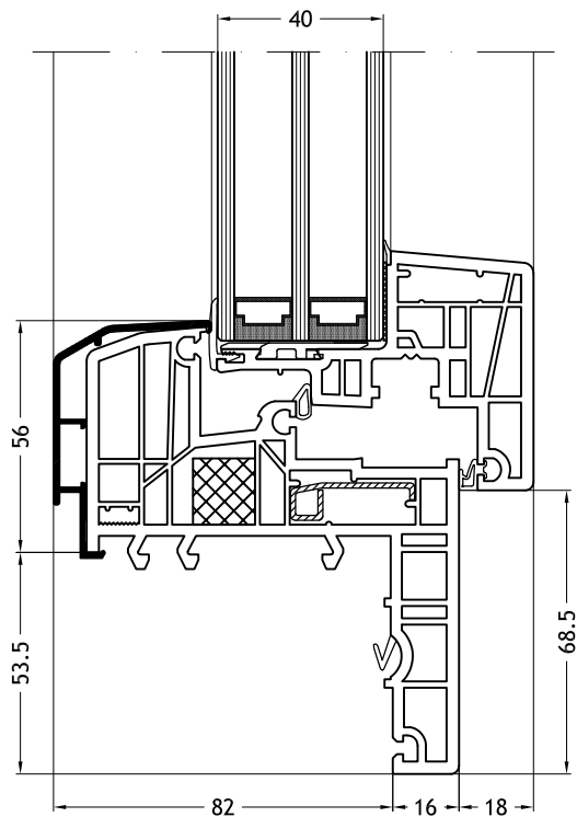
Blendrahmen Z-Form 129K mit Flügel Nova-line C 953
