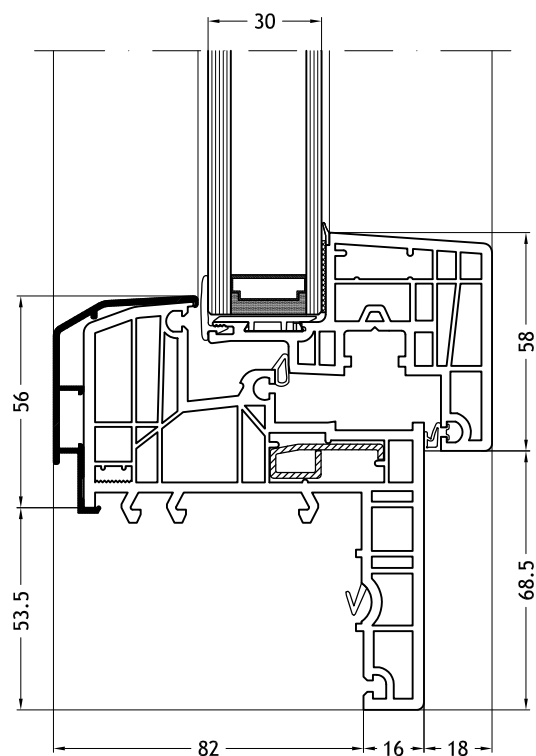
Aro em forma de Z 929K com folha Nova-line C 971
