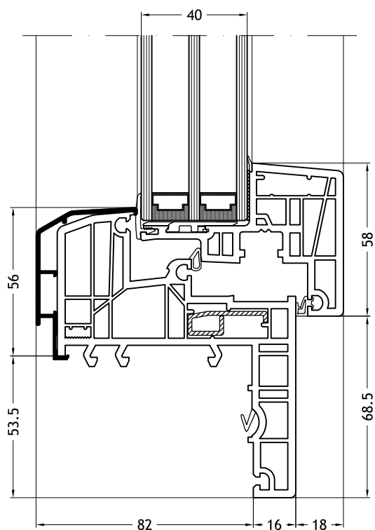
Blindraam Z-vorm 929K met vleugel Nova-line C 953
