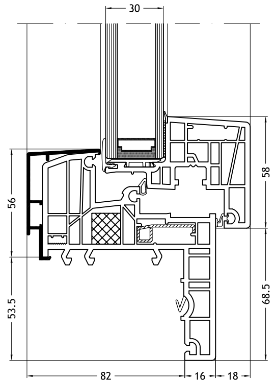
Blendrahmen Z-Form 129N mit Flügel Nova-line N 971
