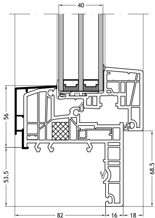
Blendrahmen Z-Form 129N mit Flügel Nova-line N 953
