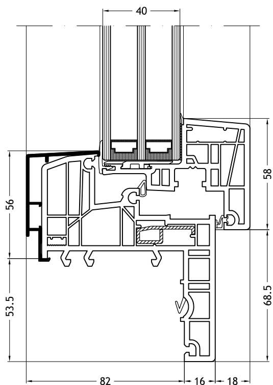
Aro em forma de Z 929N com folha Nova-line N 953
