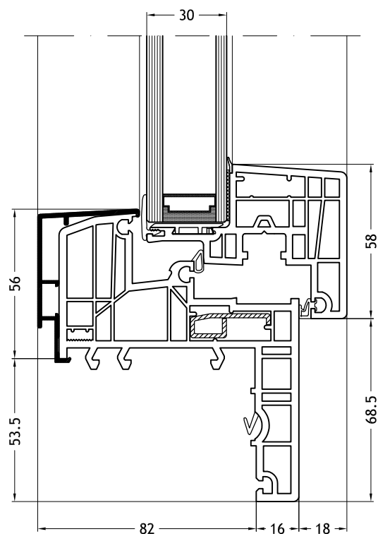
Blindraam Z-vorm 929N met vleugel Nova-line N 971
