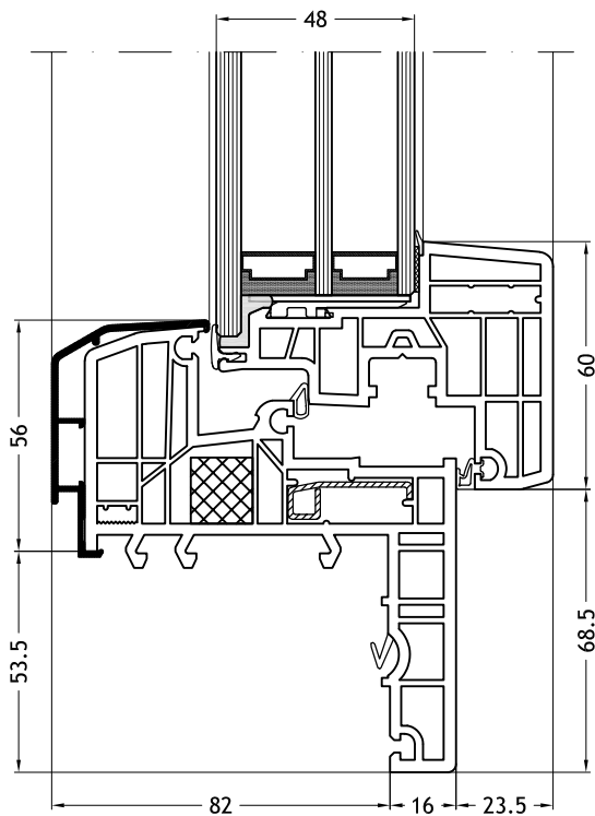
Blendrahmen Z-Form 129K mit Flügel Nova-line Plus C
