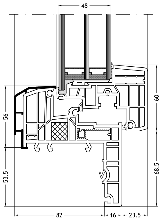
Telaio a Z 129K con anta Nova-line Plus C
