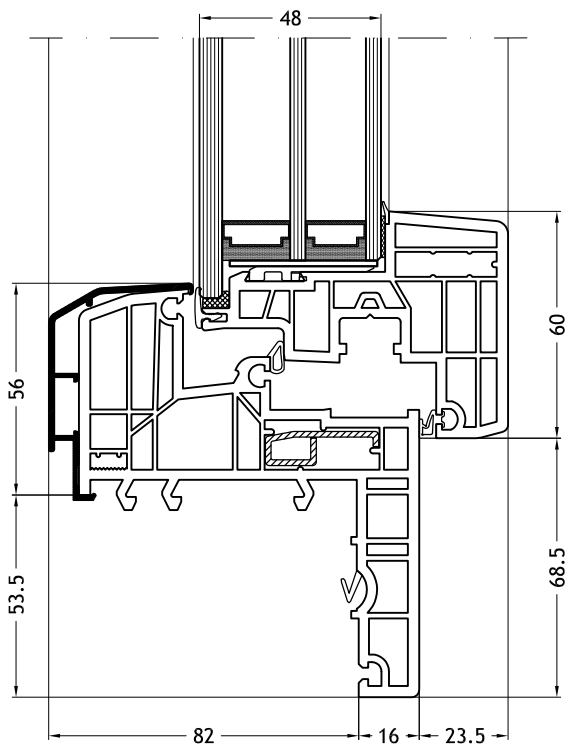
Blindraam Z-vorm 929K met vleugel Nova-line Plus C
