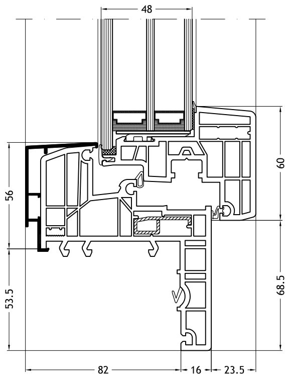
Aro em forma de Z 929N com folha Nova-line Plus N
