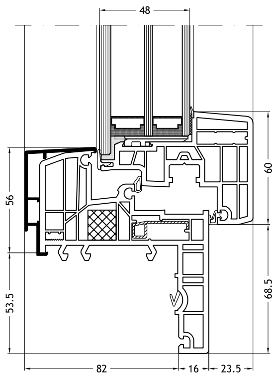
Telaio a Z 129N con anta Nova-line Plus N
