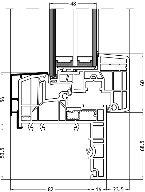
Blindraam Z-vorm 929N met vleugel Nova-line Plus N
