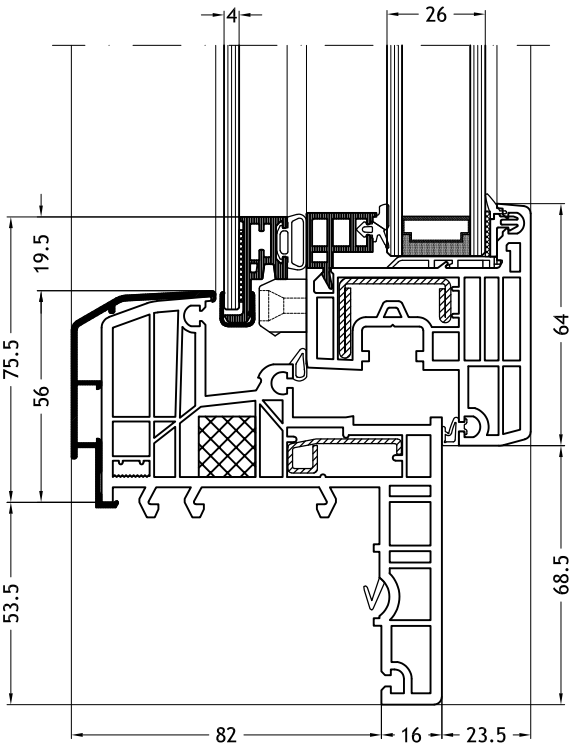
Blendrahmen Z-Form 129K mit Flügel Nova-line Twin C
