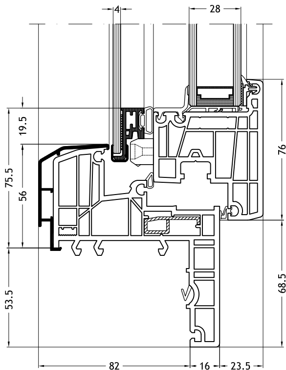
Aro em forma de Z 929K com folha Nova-line Twin C
