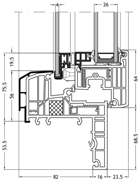
Telaio a Z 129K con anta Nova-line Twin C
