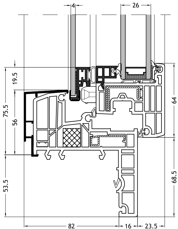
Blendrahmen Z-Form 129N mit Flügel Nova-line Twin N
