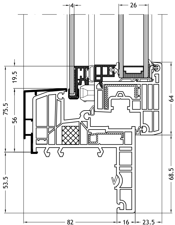
Telaio a Z 129N con anta Nova-line Twin N
