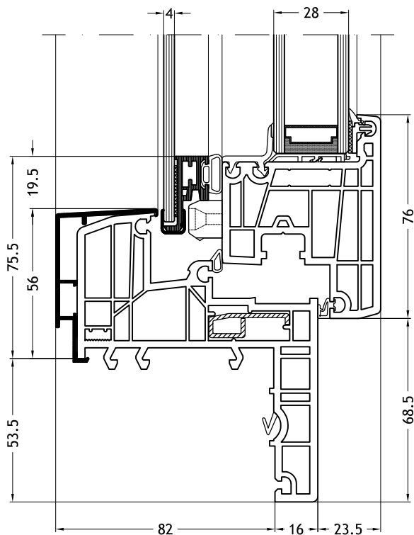
Blindraam Z-vorm 929N met vleugel Nova-line Twin N
