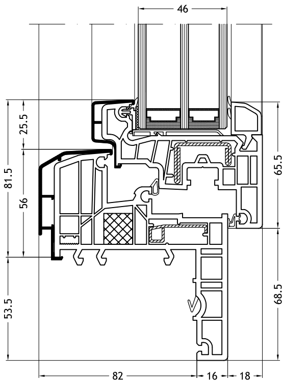
Blendrahmen Z-Form 129K mit Flügel Slim-line C
