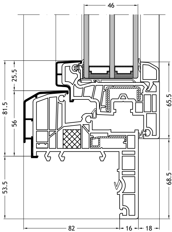
Telaio a Z 129K con anta Slim-line C
