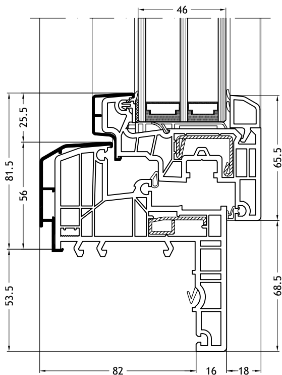
Blindraam Z-vorm 929K met vleugel Slim-line C
