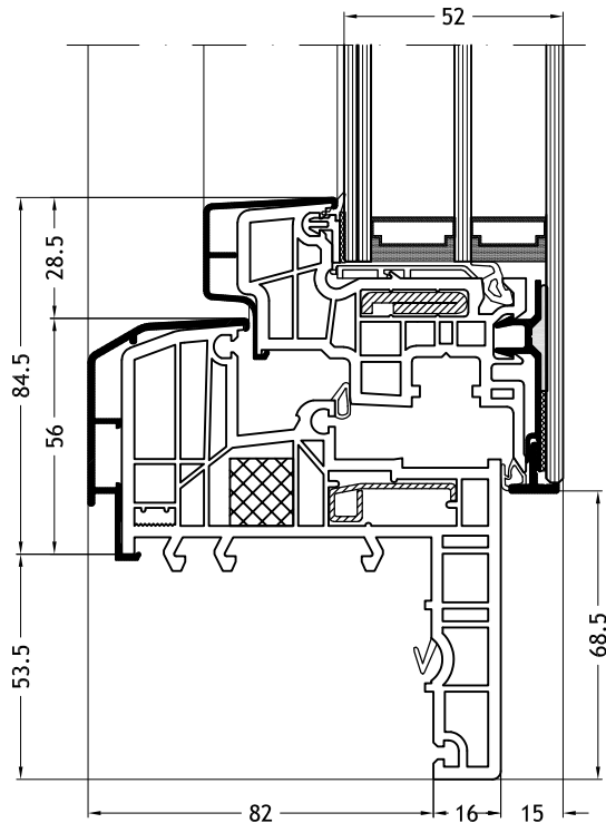
Blendrahmen Z-Form 129K mit Flügel Slim-line Cristal C
