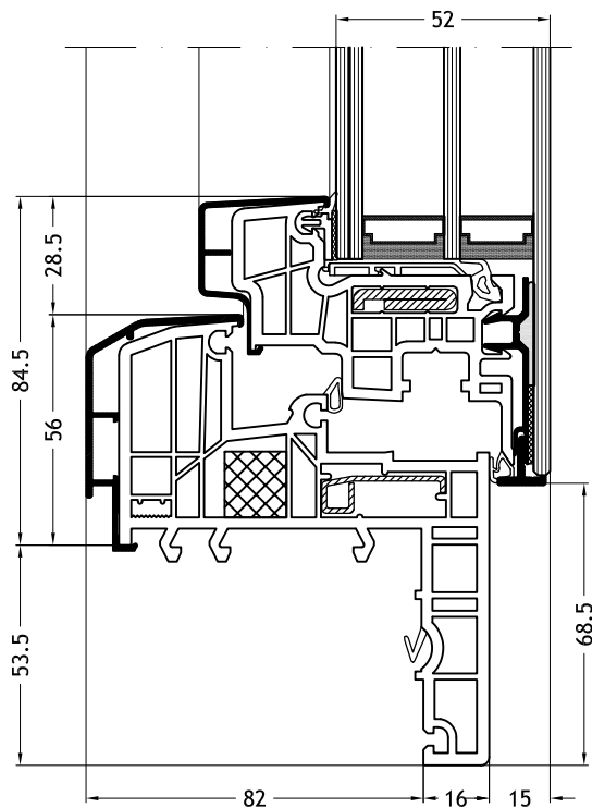
Telaio a Z 129K con anta Slim-line Cristal C
