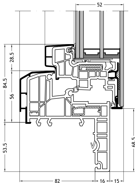
Blindraam Z-vorm 929K met vleugel Slim-line Cristal C
