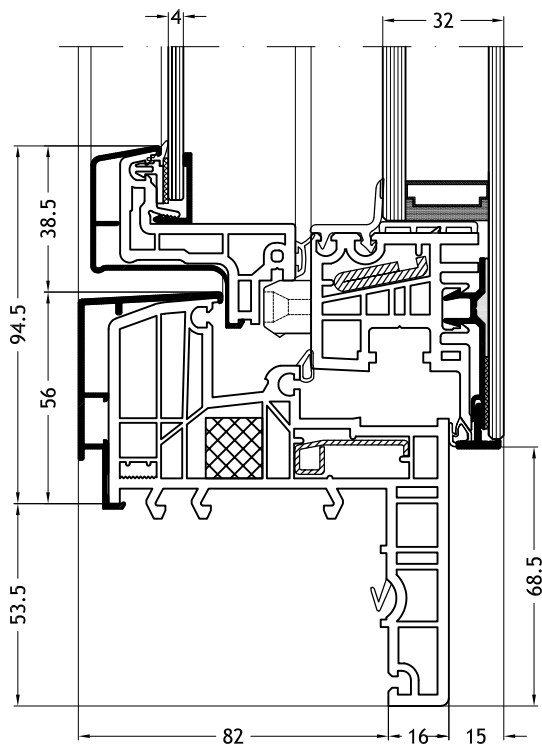
Blendrahmen Z-Form 923N mit Flügel Slim-line Cristal Twin
