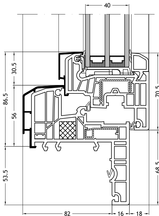
Blendrahmen Z-Form 129K mit Flügel Step-line C
