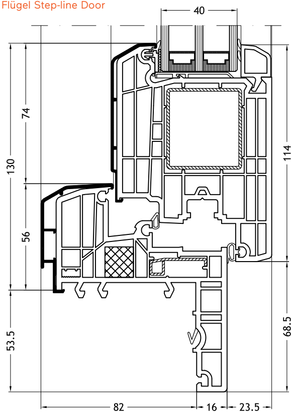
Blendrahmen Z-Form 129K mit Flügel Step-line Door
