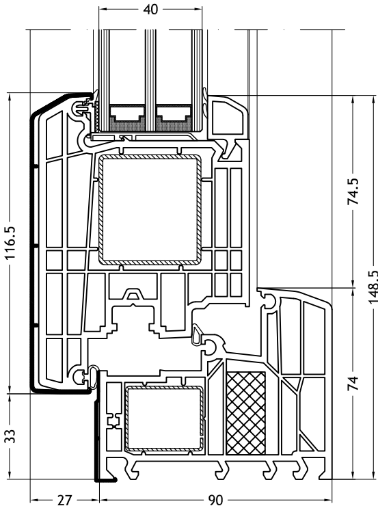
Blendrahmen L-Form A9240K mit Flügel Step-line Door out
