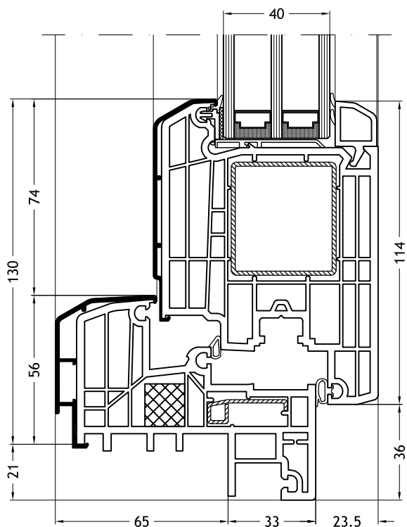
Blendrahmen Z-Form 923K mit Flügel Step-line Door
