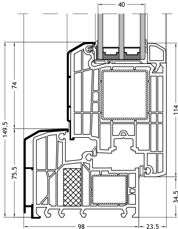
Blendrahmen L-Form 924K mit Flügel Step-line Door
